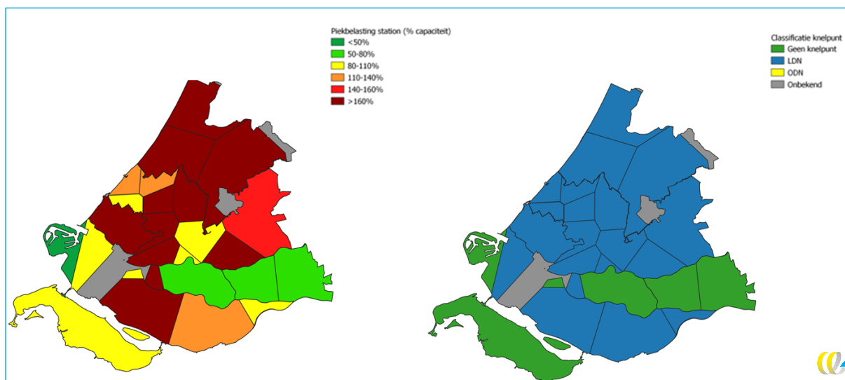
Figuur 70 - Visualisatie overbelasting koppelpunten scenario 2050 Internationale Sturing zonder flex
