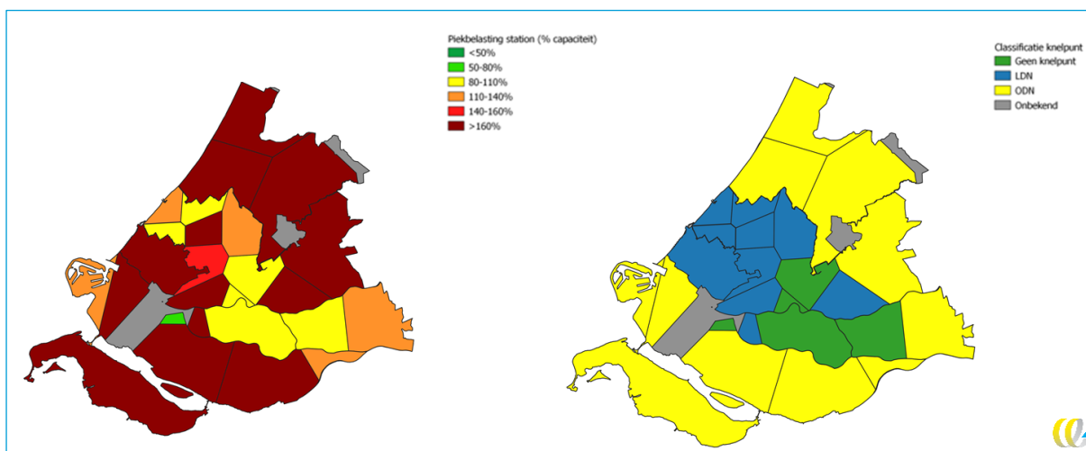
Figuur 64 - Visualisatie overbelasting koppelpunten scenario 2050 Regionale Sturing zonder flex
