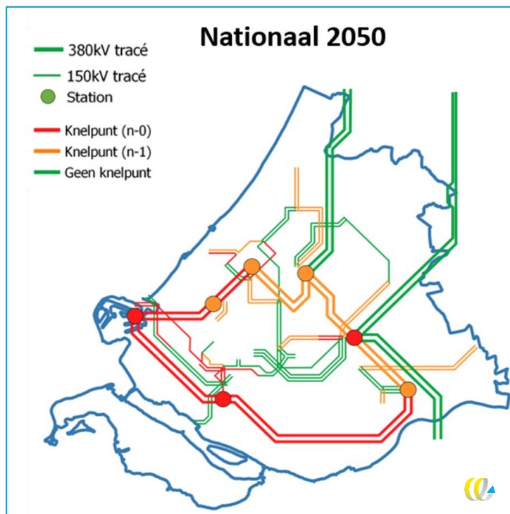
Figuur 60 - Visualisatie overbelasting hoogspanningsnet 2050 Nationale Sturing-scenario
