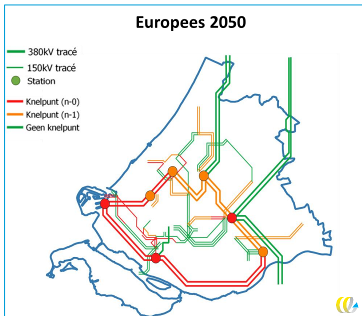
Figuur 61 - Visualisatie overbelasting hoogspanningsnet 2050 Europese Sturing-scenario
