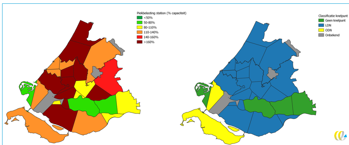
Figuur 68 - Visualisatie overbelasting koppelpunten scenario 2050 Europese Sturing zonder flex
