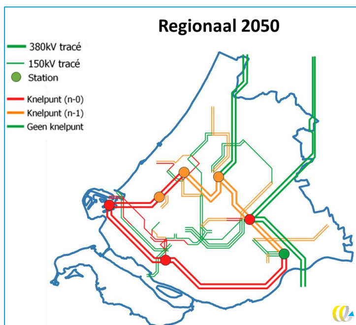
Figuur 59 - Visualisatie overbelasting hoogspanningsnet 2050 Regionale Sturing-scenario
