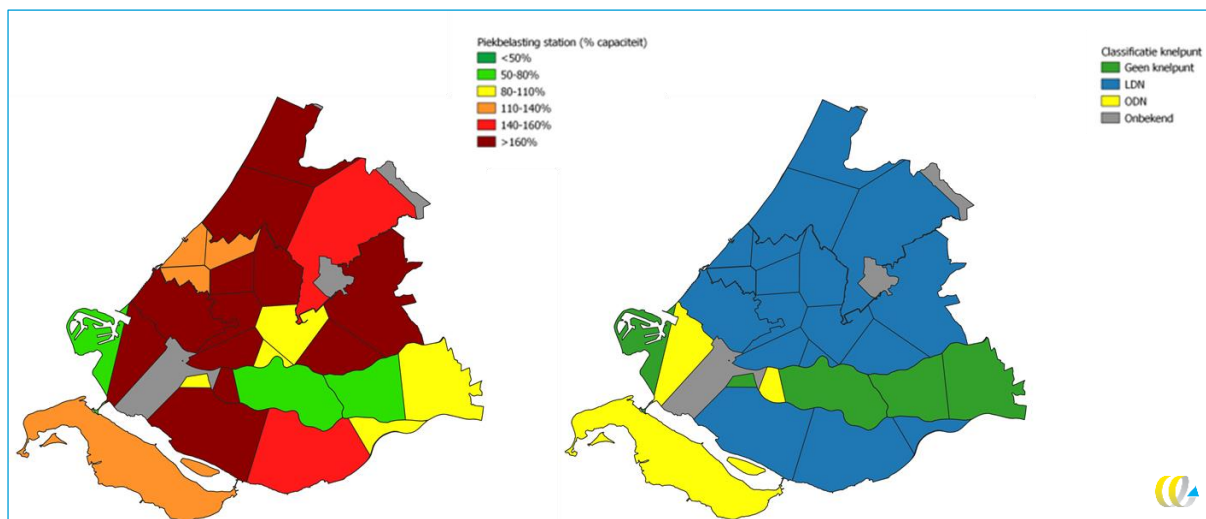
Figuur 67 - Visualisatie overbelasting koppelpunten scenario 2050 Nationale Sturing met flex
