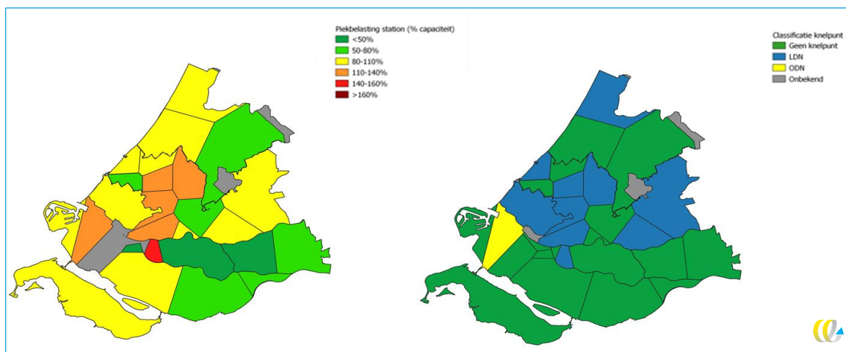
Figuur 63 - Visualisatie overbelasting koppelpunten scenario 2030 Klimaatakkoord
