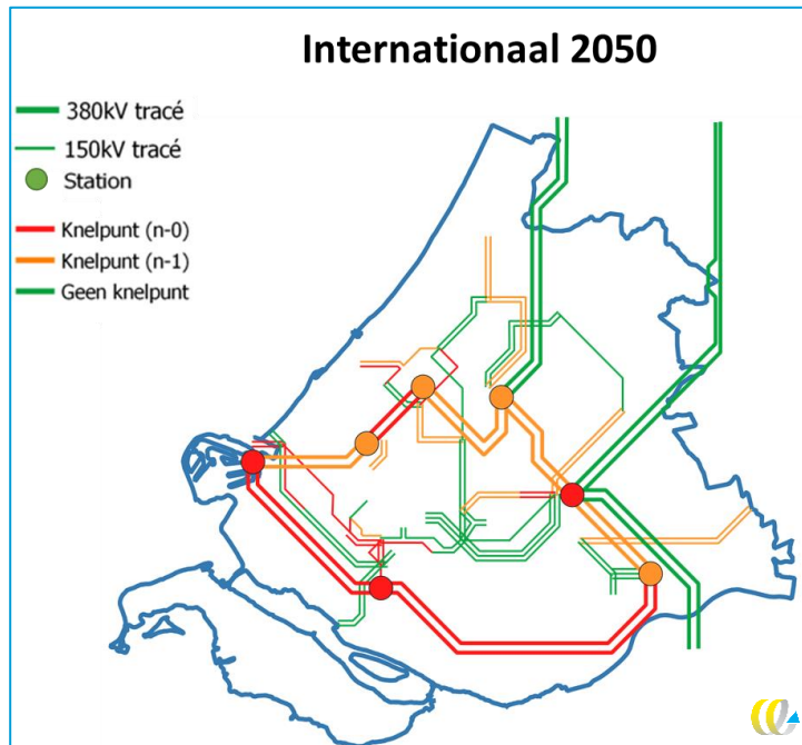
Figuur 62 - Visualisatie overbelasting hoogspanningsnet 2050 Internationale Sturing-scenario
