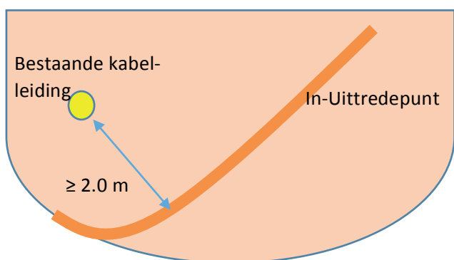
Dwarsdoorsnede
